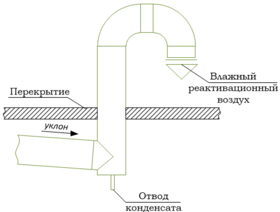
Рисунок 4.9 – Пример прокладки вертикального воздуховода выбросного реаквационного воздуха
