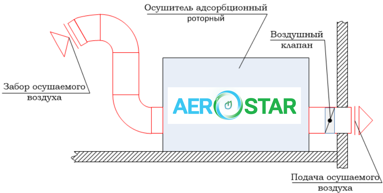
Рисунок 4.10 – Пример прокладки воздухопроводов осушаемого воздуха
